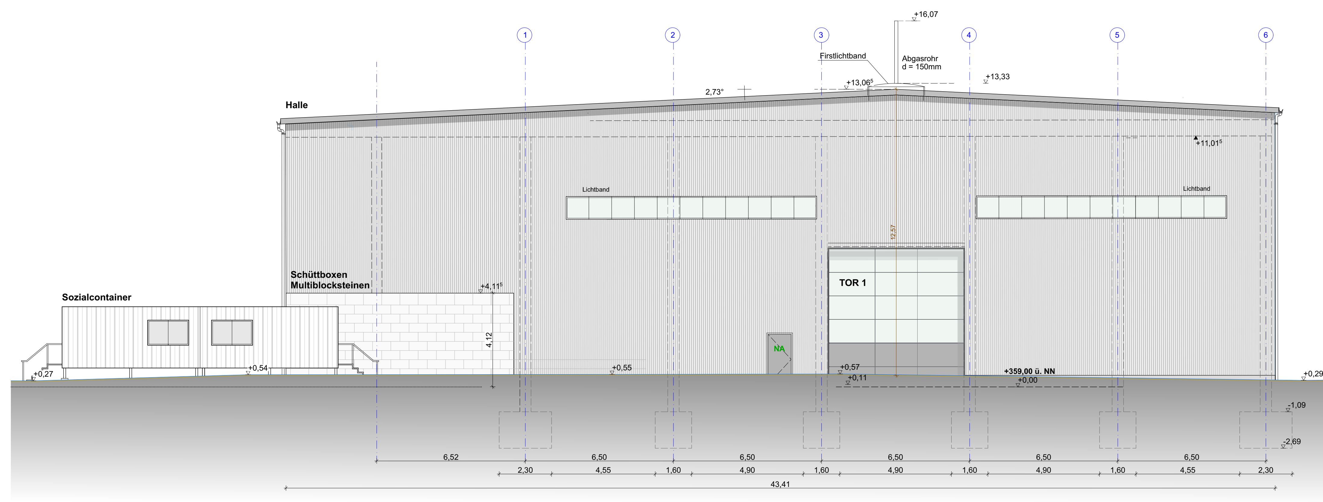
ANSICHT 7 (HALLE NORD)
