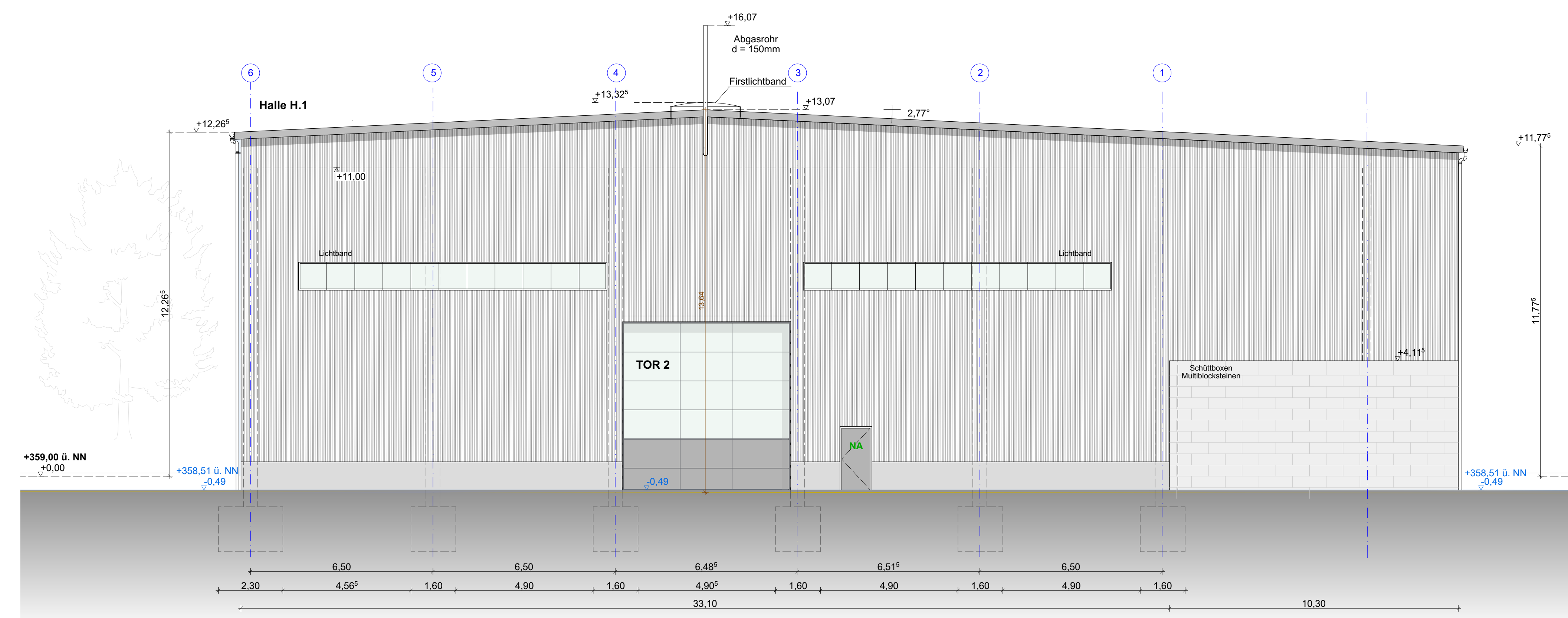
ANSICHT 8 (HALLE SÜD)
